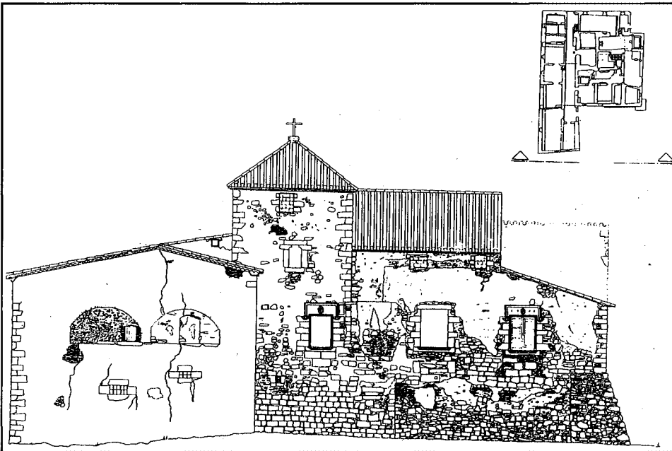
Il·lustració 6 Arcadi Pla Masmiquel, arquitecte Plànol de l'aixecament de l'estat actual del Mas Barril. Façana sud.
