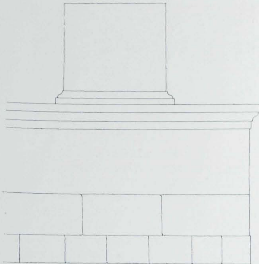
Fig. 27. — Motlluratje del basament y dels pedestals Escala 1:20
