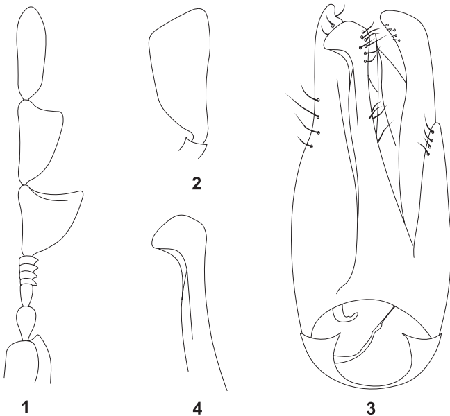
Figures 1-4. Dorcatoma (Dorcatoma) punctulata : 1. antena del mascle; 2. últim artell dels palps maxil·lars; 3. eedeagus; 4. detall de la peça mitjana del eedeagus.
